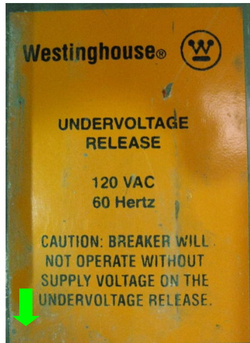
NON-OEM
